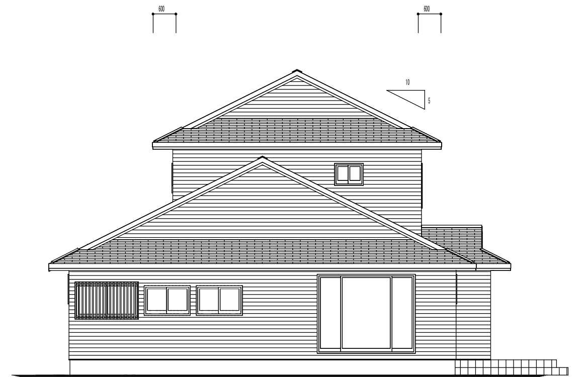
西立面图 1/100
