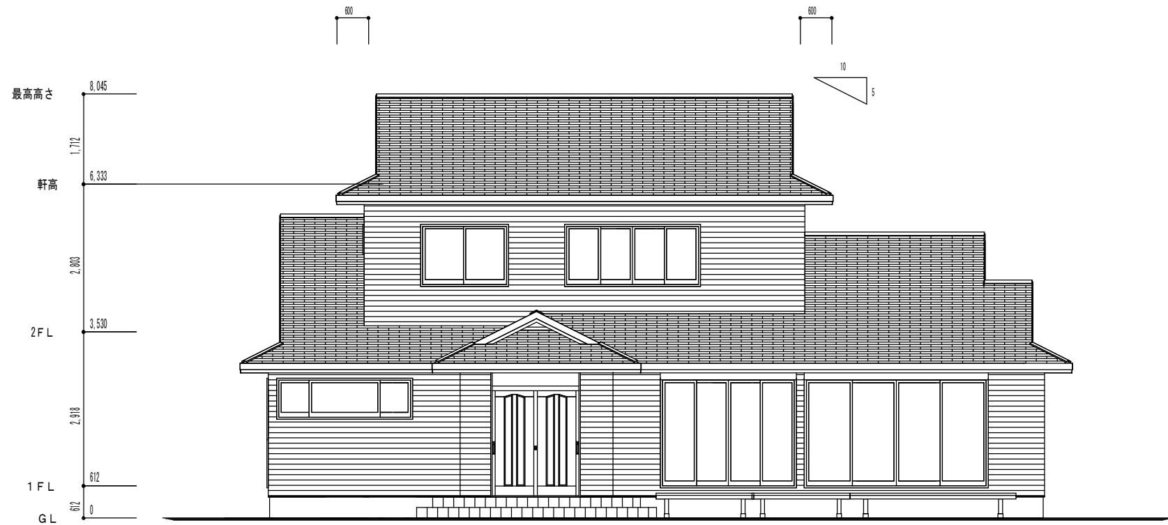
南立面图 1/100
