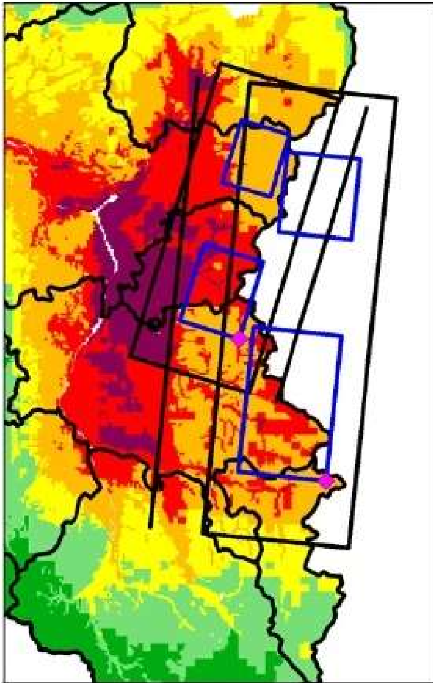
図2 横手盆地真昼山連動の震度分布図拡大図(図1青枠内)
