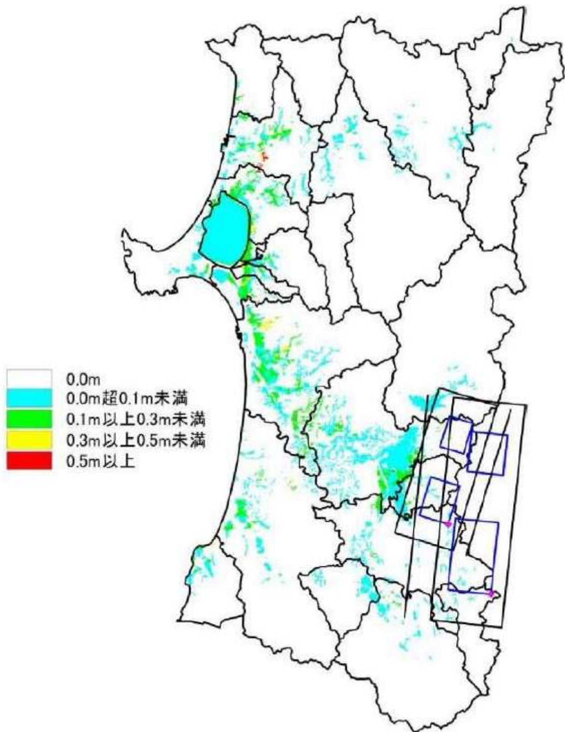
図4 横手盆地真屋山連動の液状化による沈下量図
