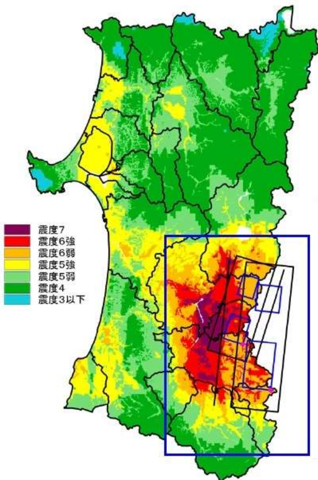
図1 横手盆地真昼山連動の震度分布図(詳細法)
