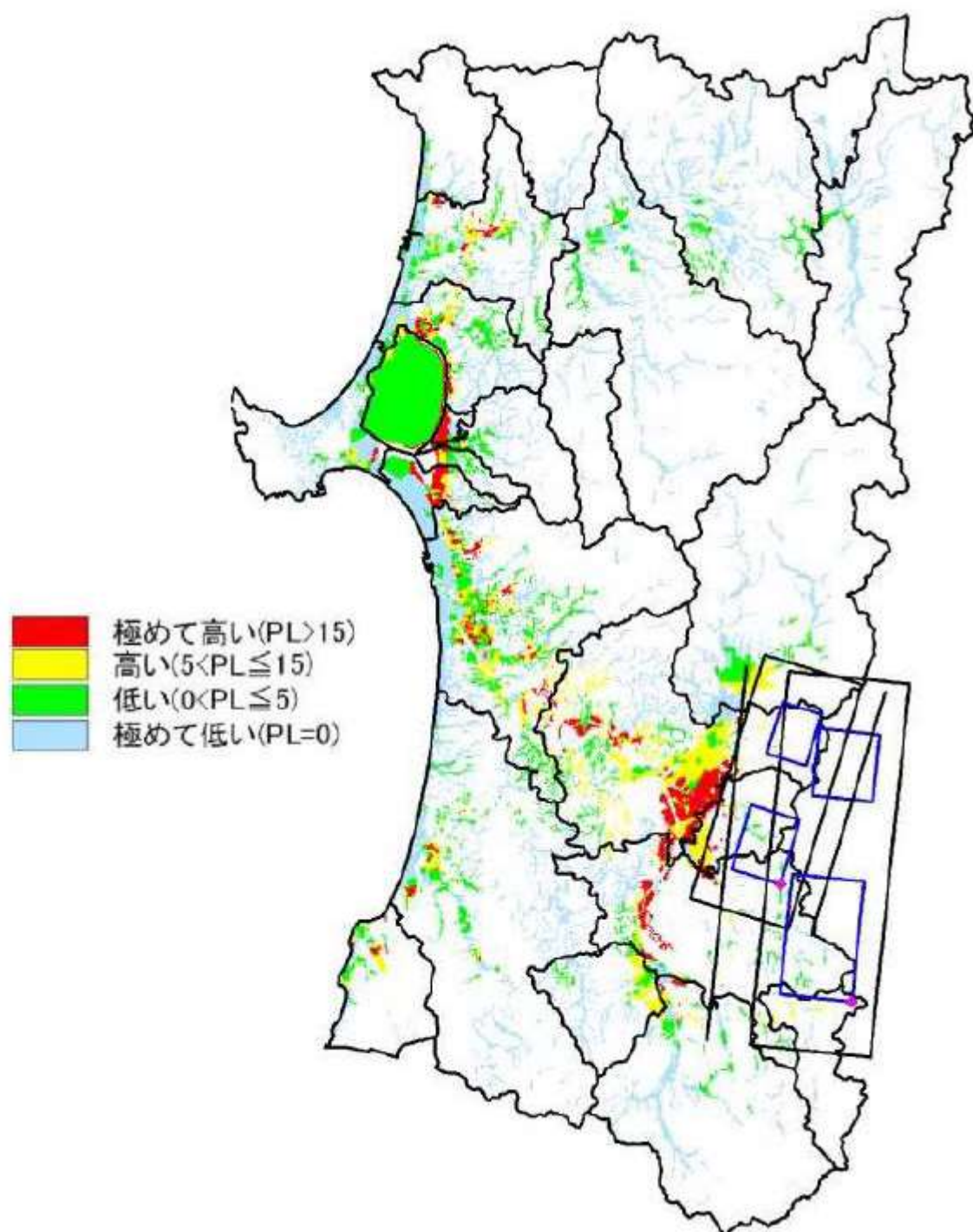
図3 横手盆地真昼山連動の液状化危険度分布図
