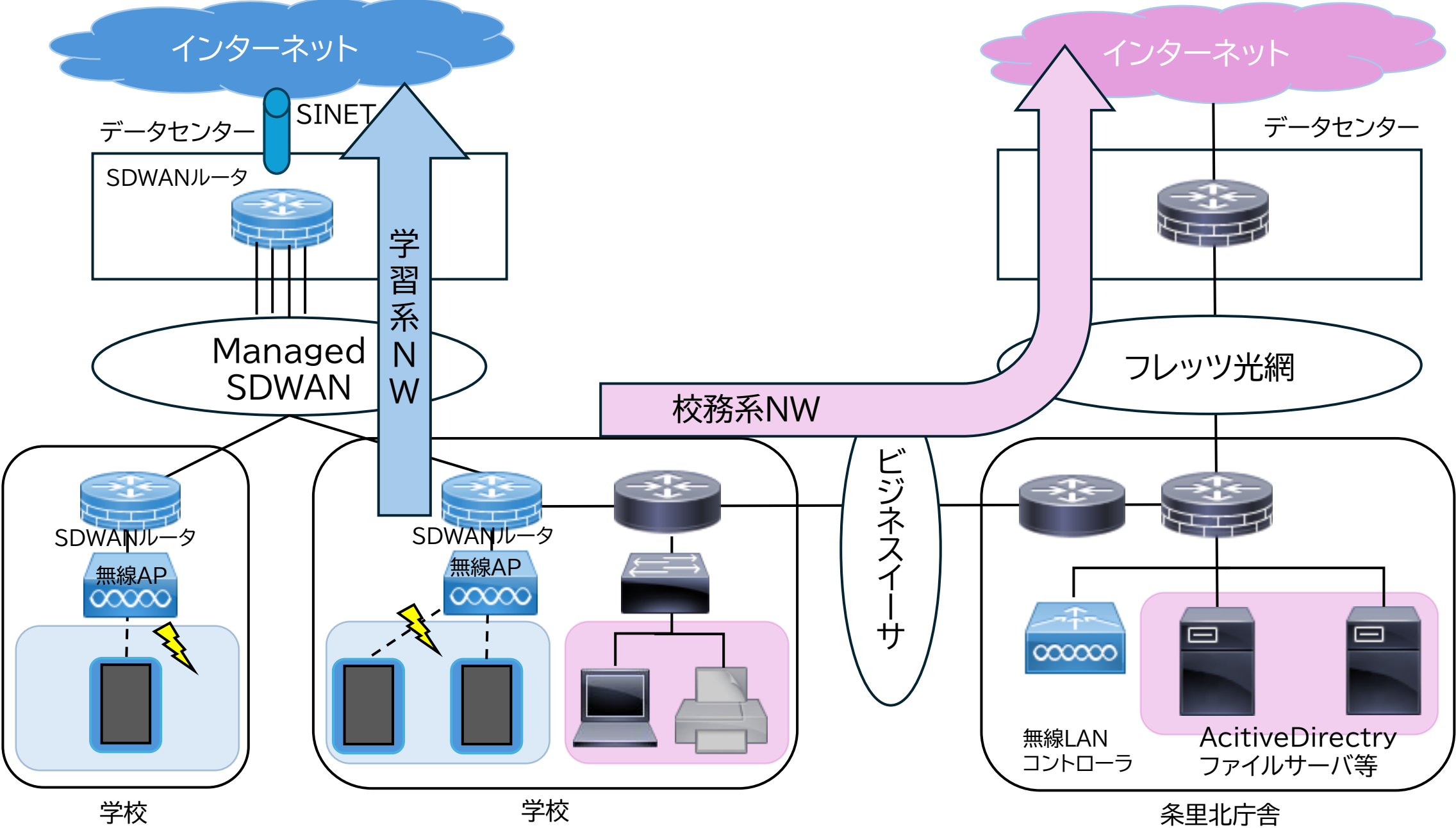
資料1:ネットワーク構成図
