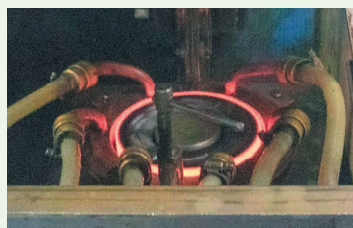
▲高周波の電磁誘導で部品の表面を加熱し、強度を上げる『高周波焼入装置』
