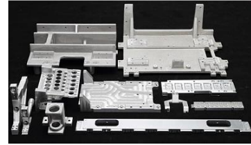
▲ 吉野工場の精密機械加工部品
