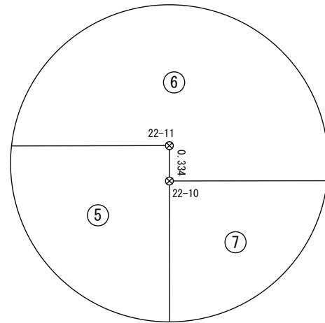
拡大図 (C) S=1:50
