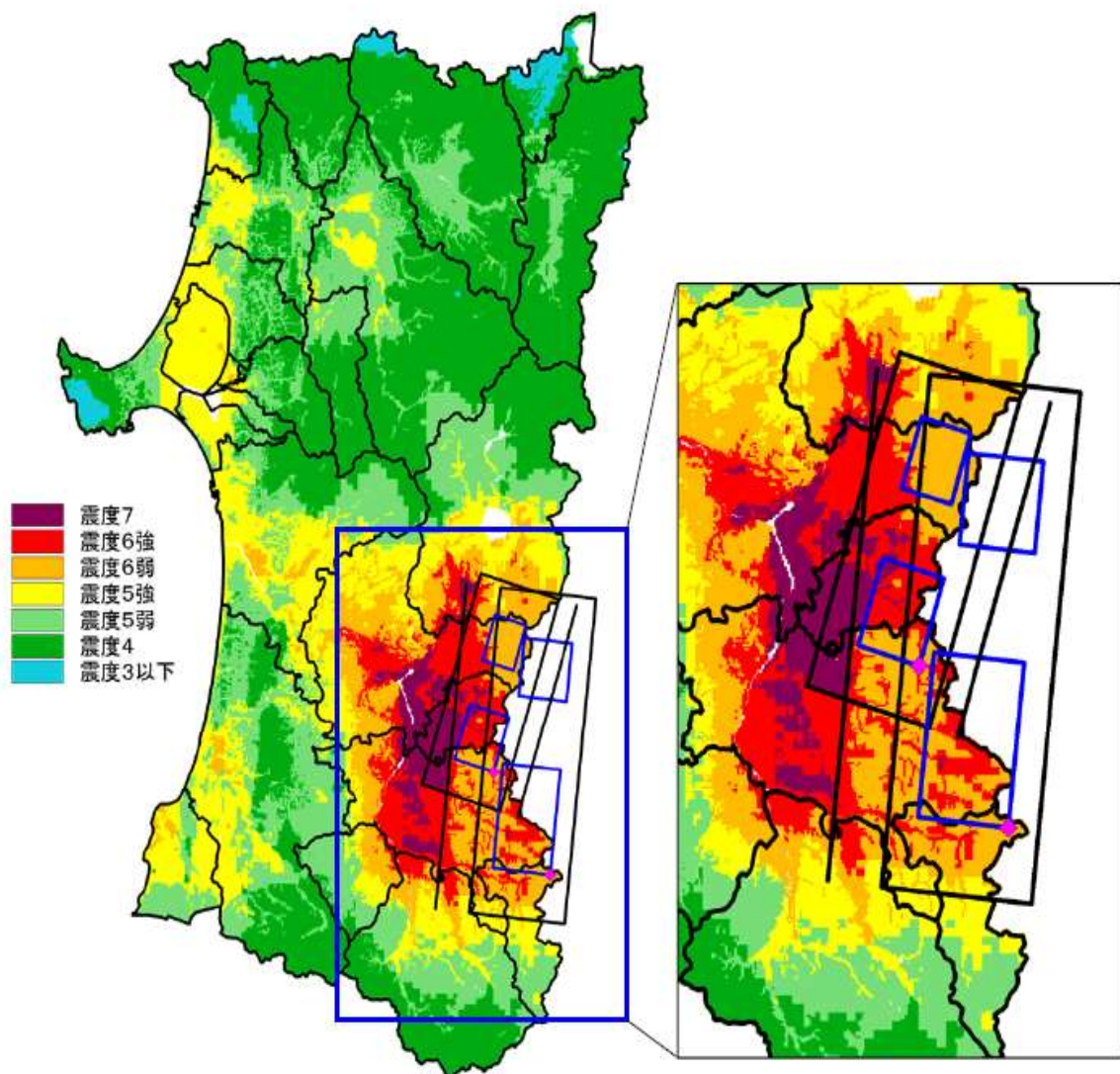
図-4.5.13 震度分布図(詳細法) (青枠：アスペリティの位置、ひし形：破壊開始点の位置)
