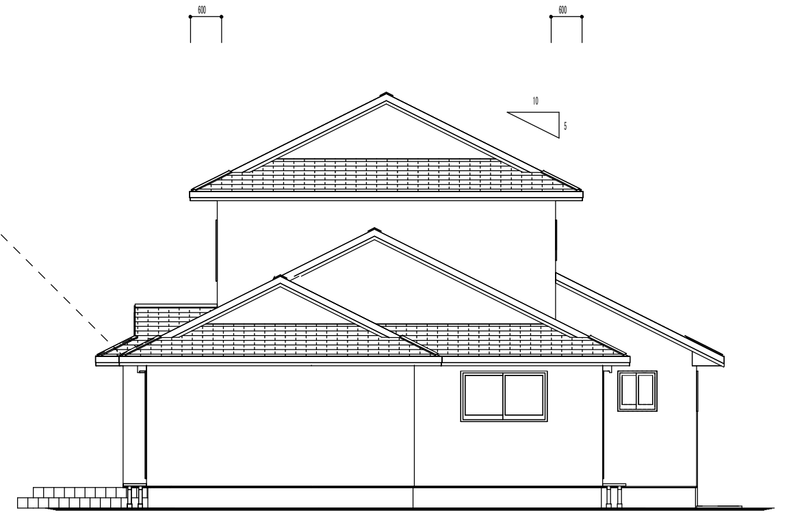
東立面図 1/100
