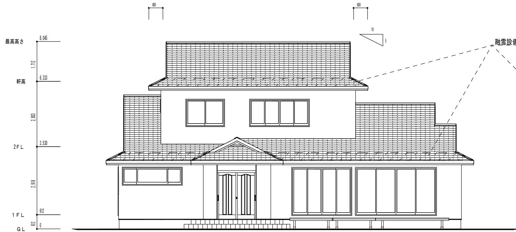
南立面図 1/100
