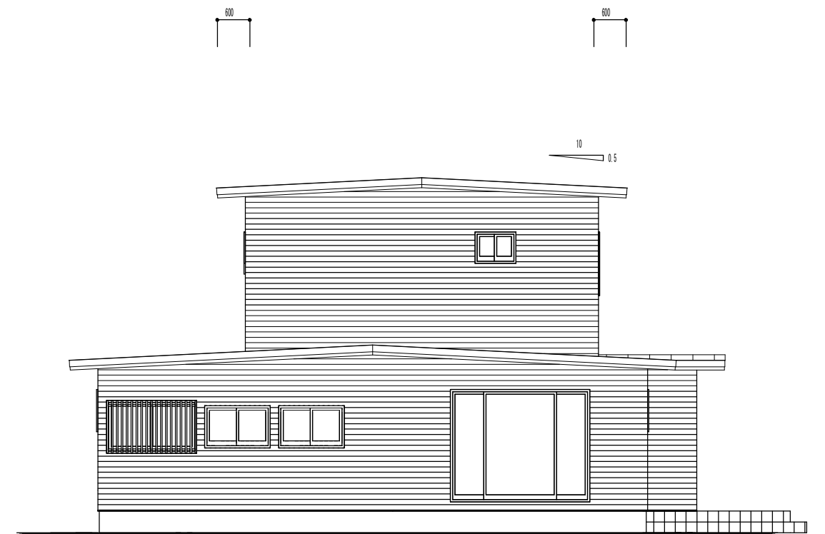
西立面图 1/100
