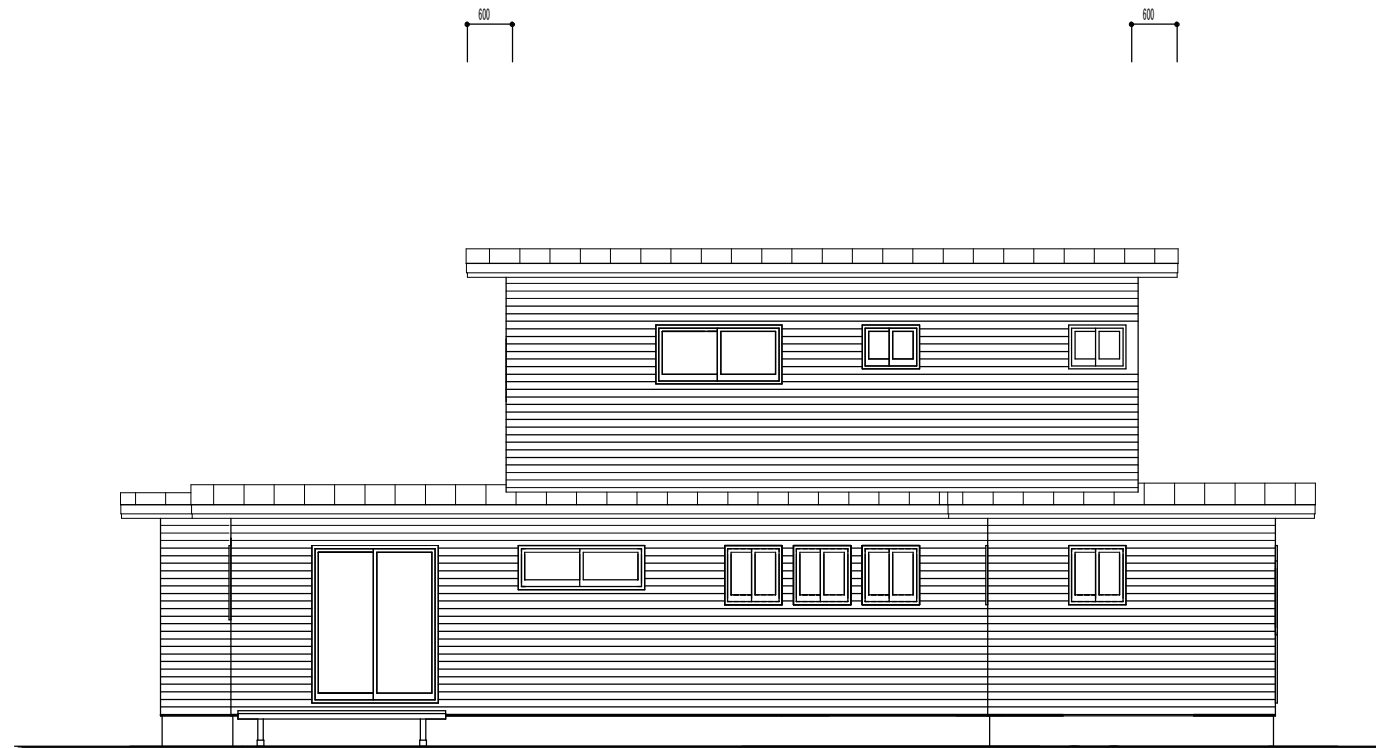
北立面图 1/100
