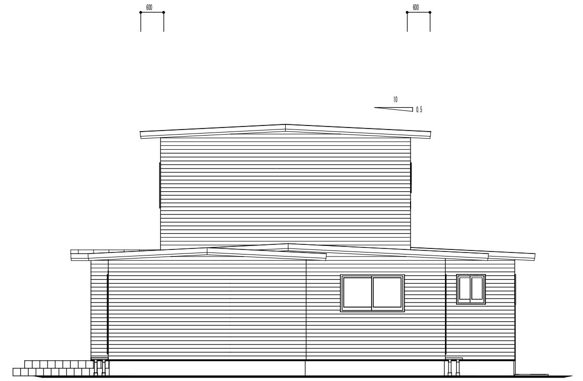
東立面图 1/100
